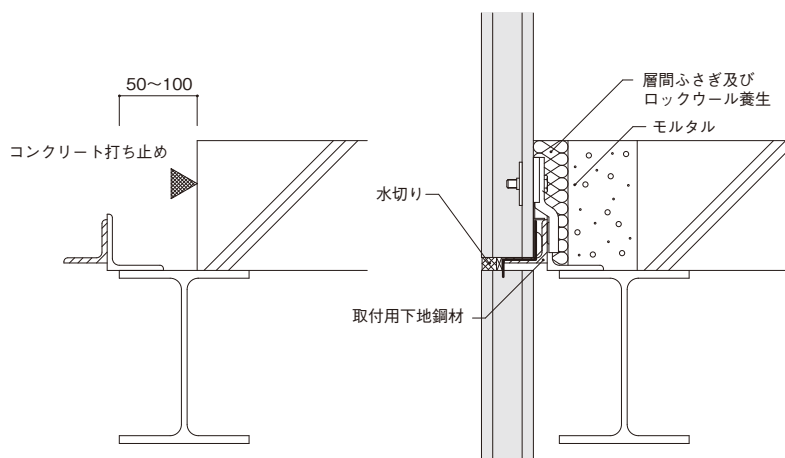
図8 スラブ止め位置
