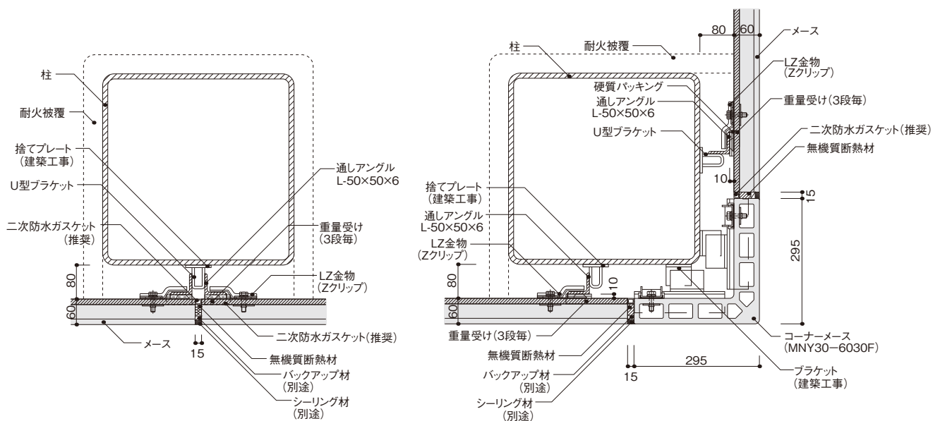
水平断面図
