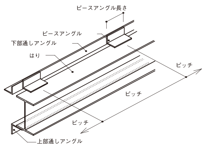
図4 下地取付図
