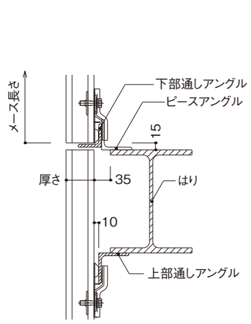
図3 断面詳細図
