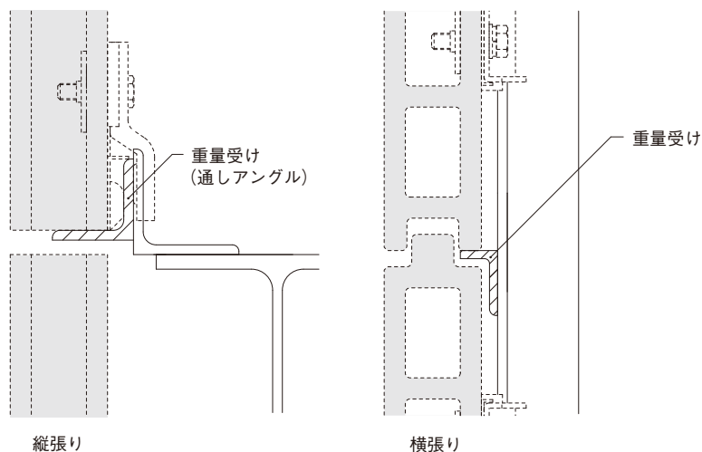
図12 重量受け
