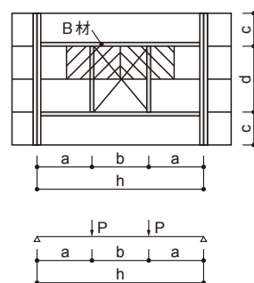
横材(B材)
