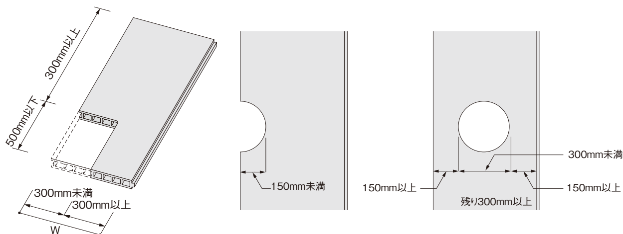
図7 メースの孔あけ及び切り込みの限度
