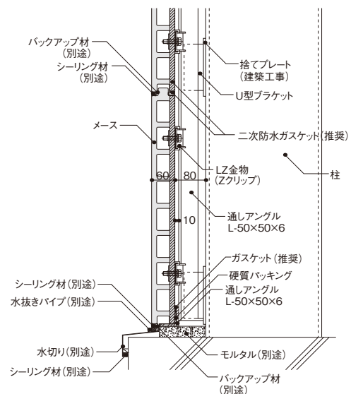
垂直断面図
