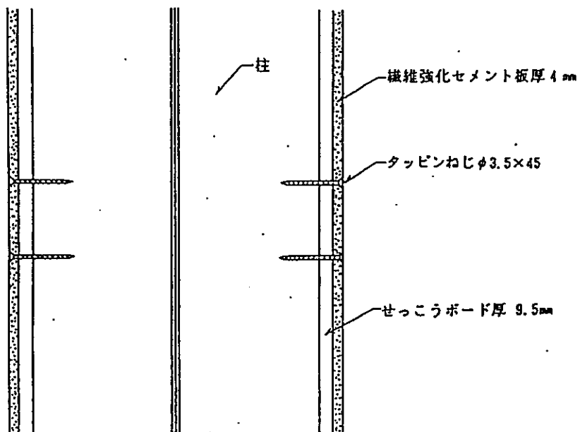
垂直断面図
