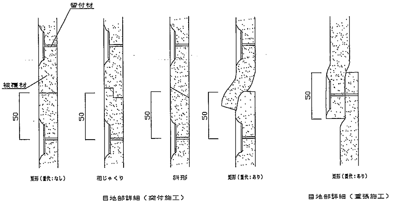
図3 構造説明図
