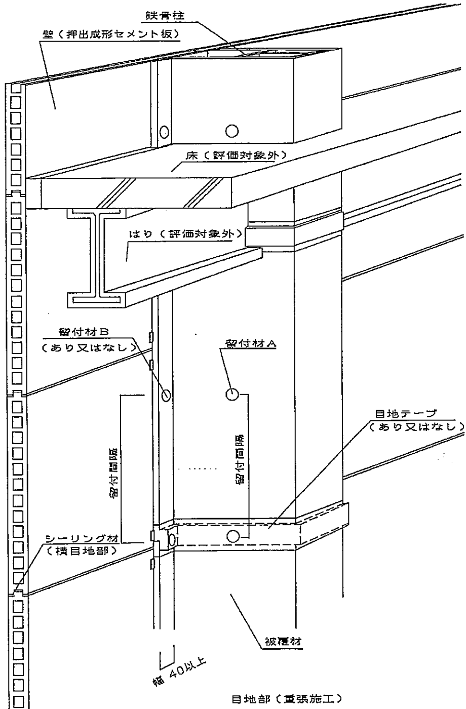
図2 構造説明図
