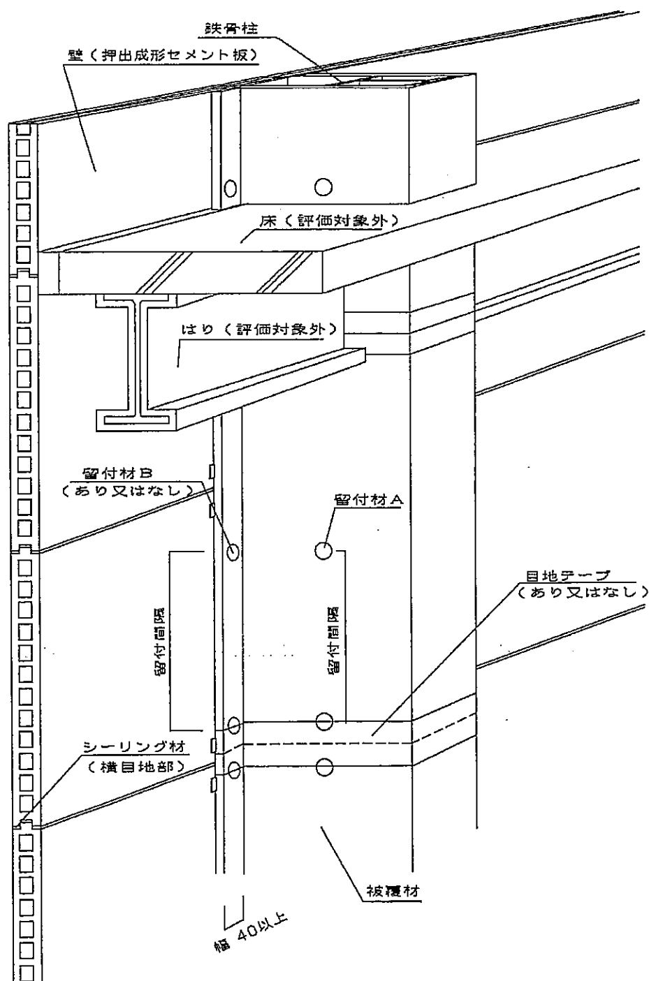
目地部 (突付施工)
