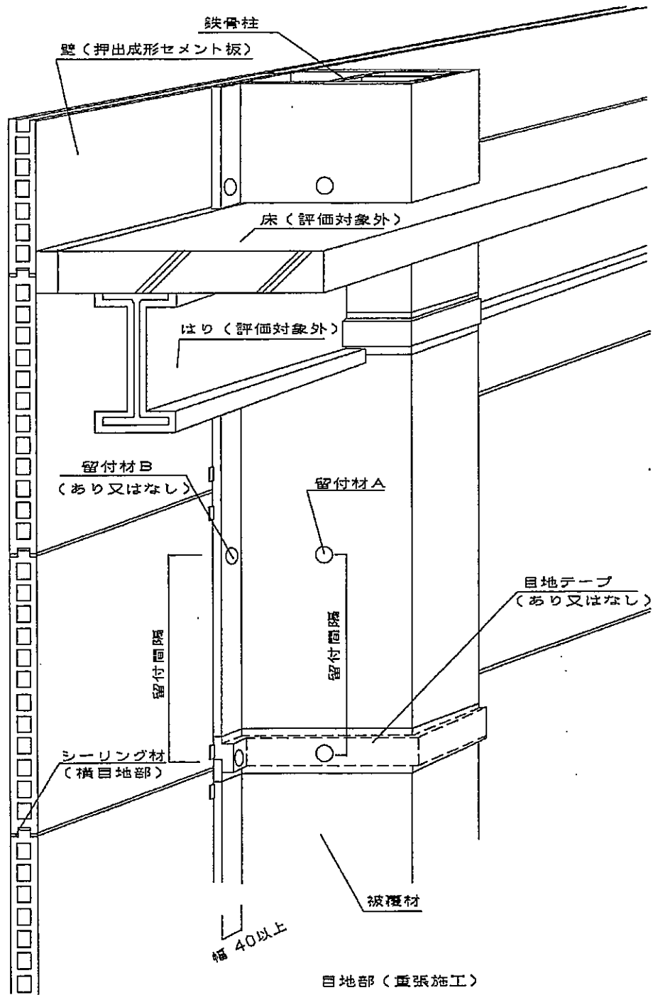
図5 施工図
