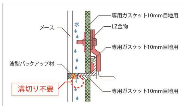
縦張り工法 断面図
