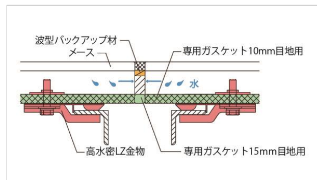
横張り工法 平面図
