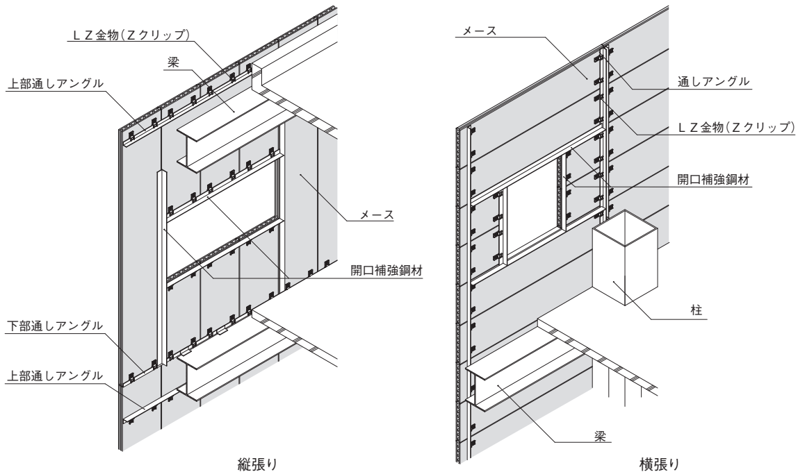
図13 開口補強
