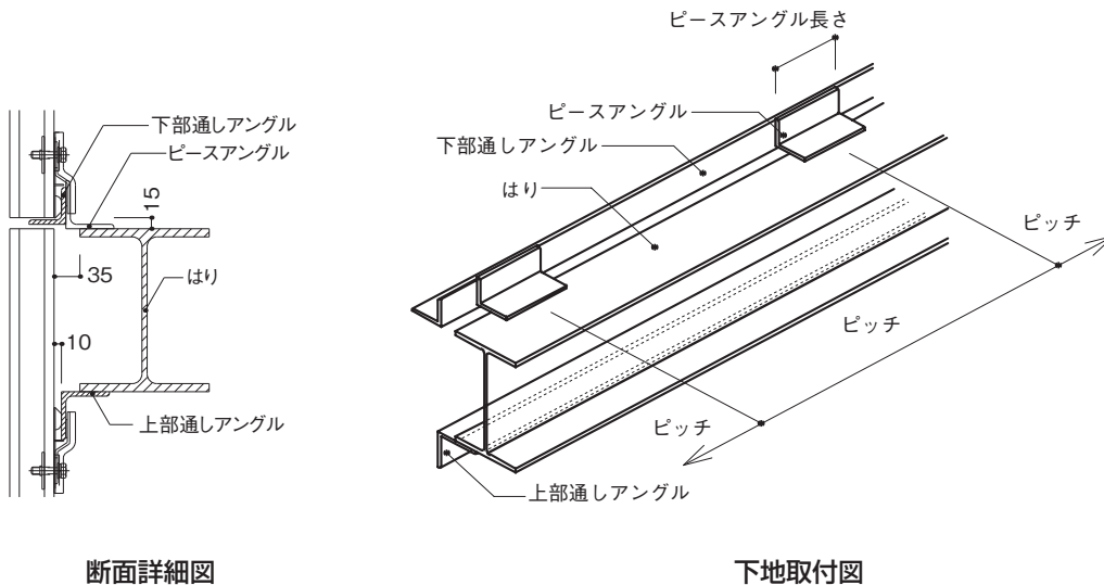
断面詳細図
