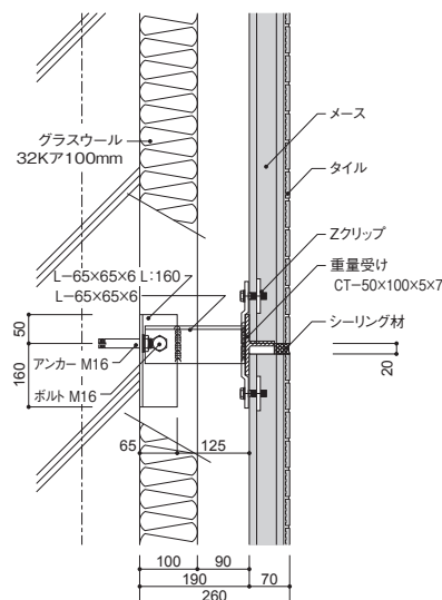
(断面詳細図)
