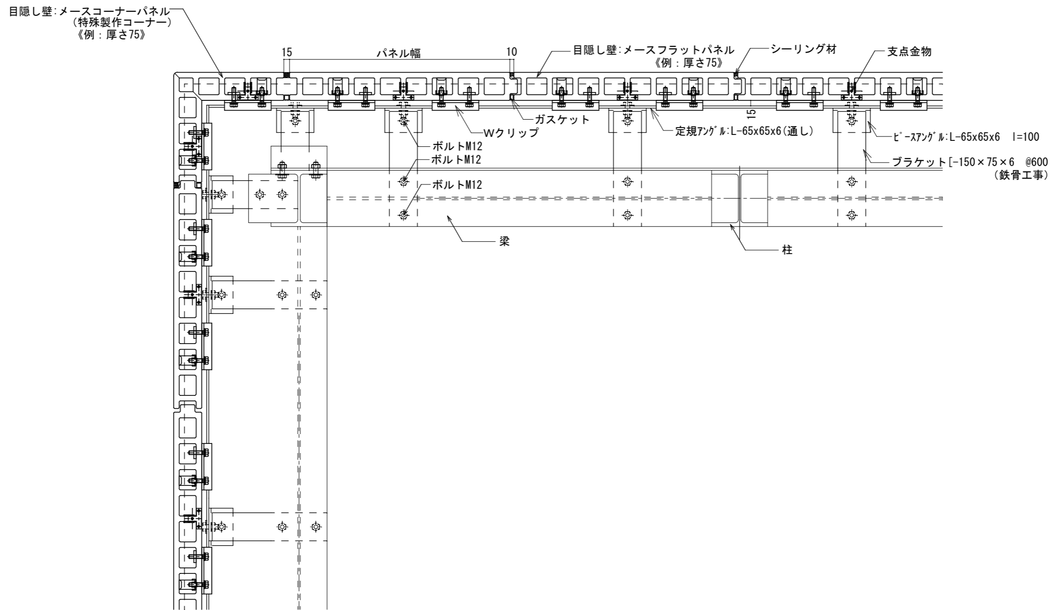
水平断面詳細図
