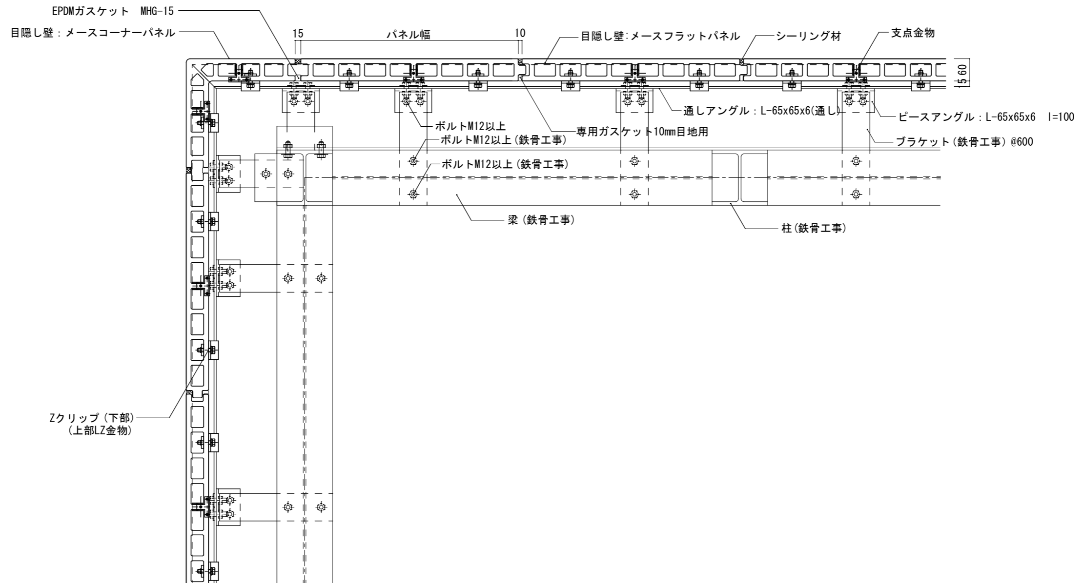
水平断面詳細図
